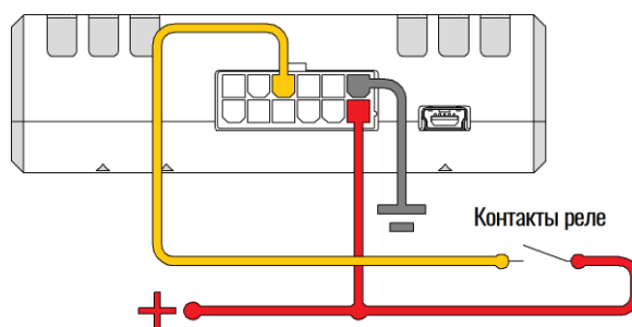
Рисунок 2.11 Варианты подключения дискретных датчиков
