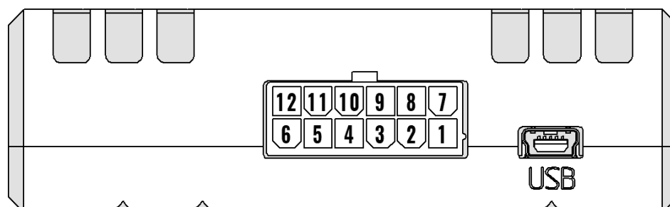
Рисунок 2.2 Нумерация выводов УМКа314х
