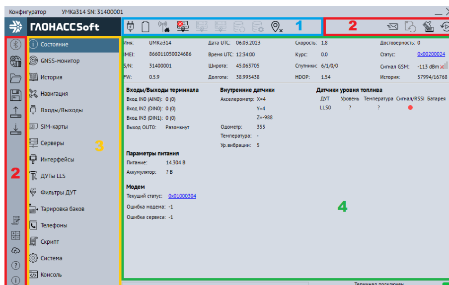
Рисунок 3.22 Стартовое окно «Состояние»
