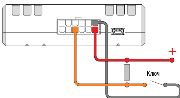
Рисунок 2.8 Подключение с подтяжкой к «+»
