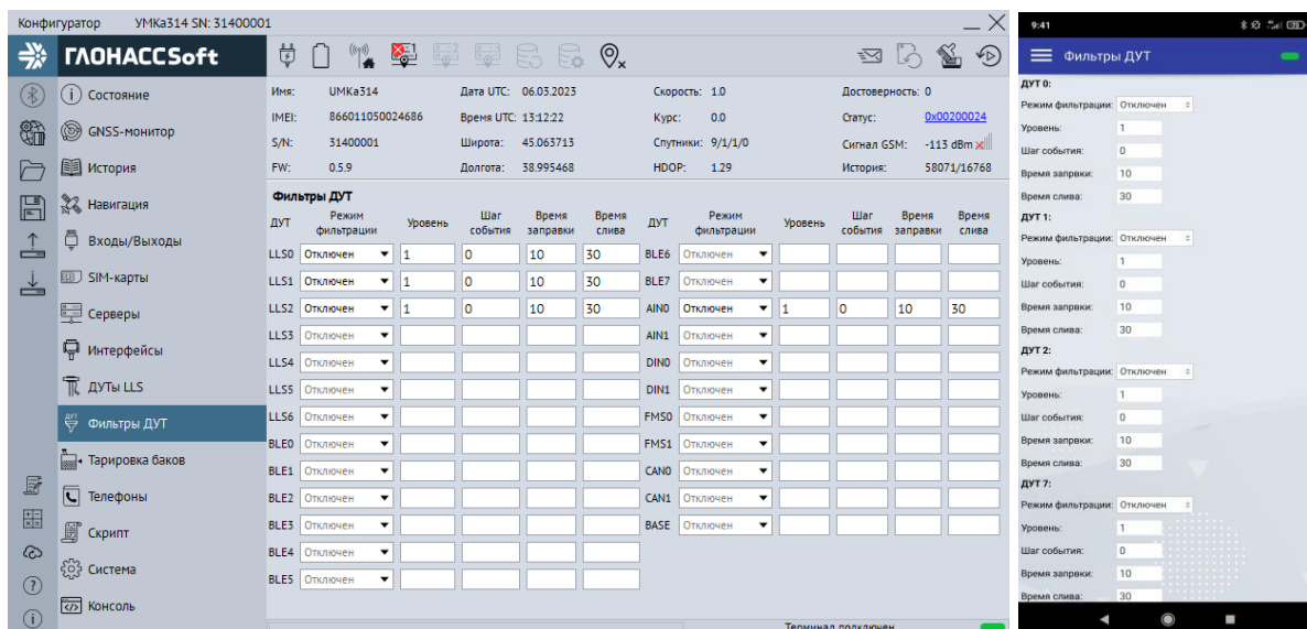
Рисунок 3.38 Вкладка «Фильтры ДУТ»
