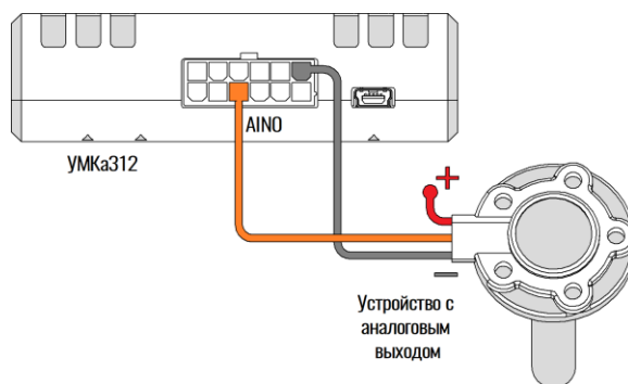
Рисунок 2.7 Подключение аналоговых источников
