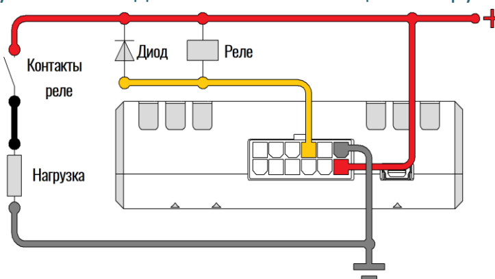
Рисунок 2.13 Подключение мощной нагрузки
