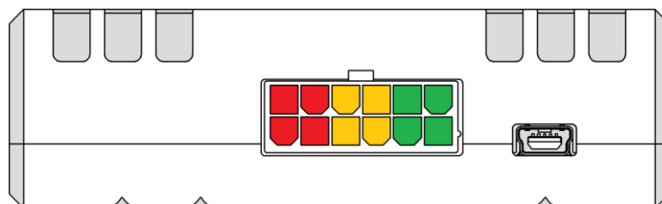
Рисунок 3.15 Расположение индицирующих светодиодов
