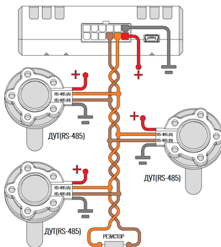
Рисунок 2.14 Подключение ДУТ по интерфейсу RS-485
