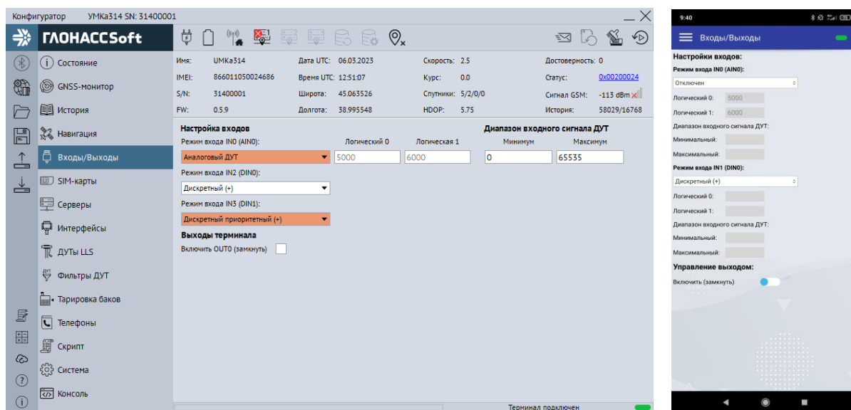
Рисунок 3.33 Вкладка «Входы/Выходы»
