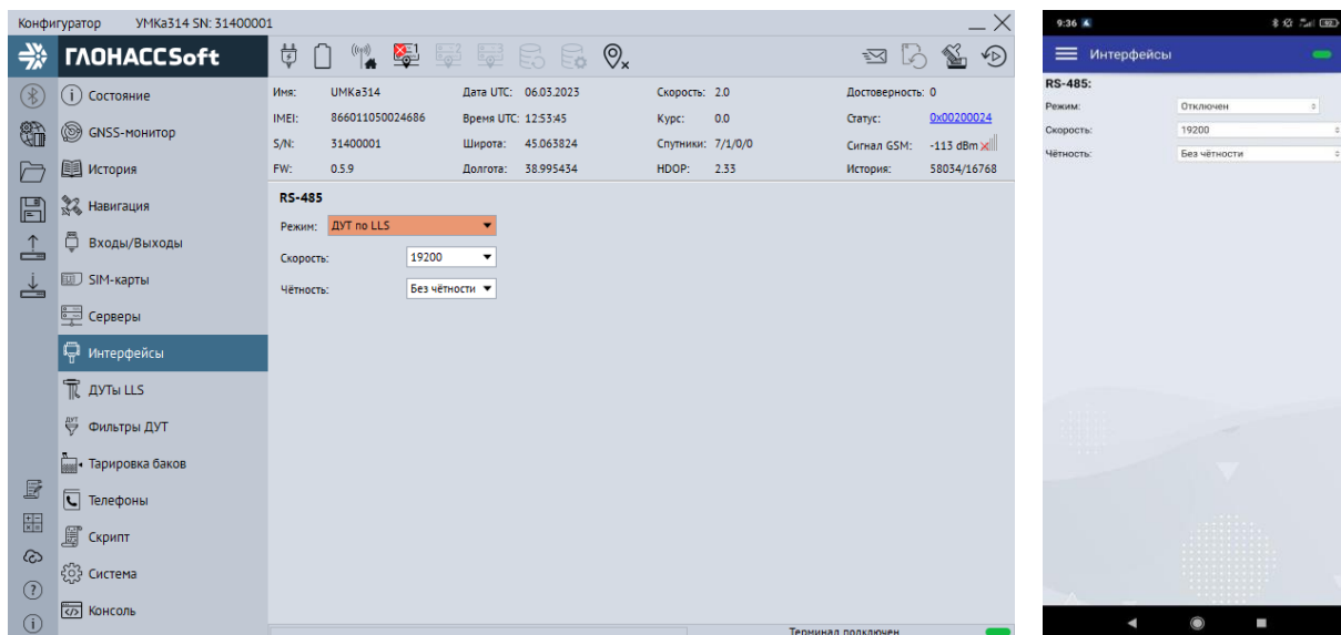
Рисунок 3.36 Вкладка «Интерфейсы»
