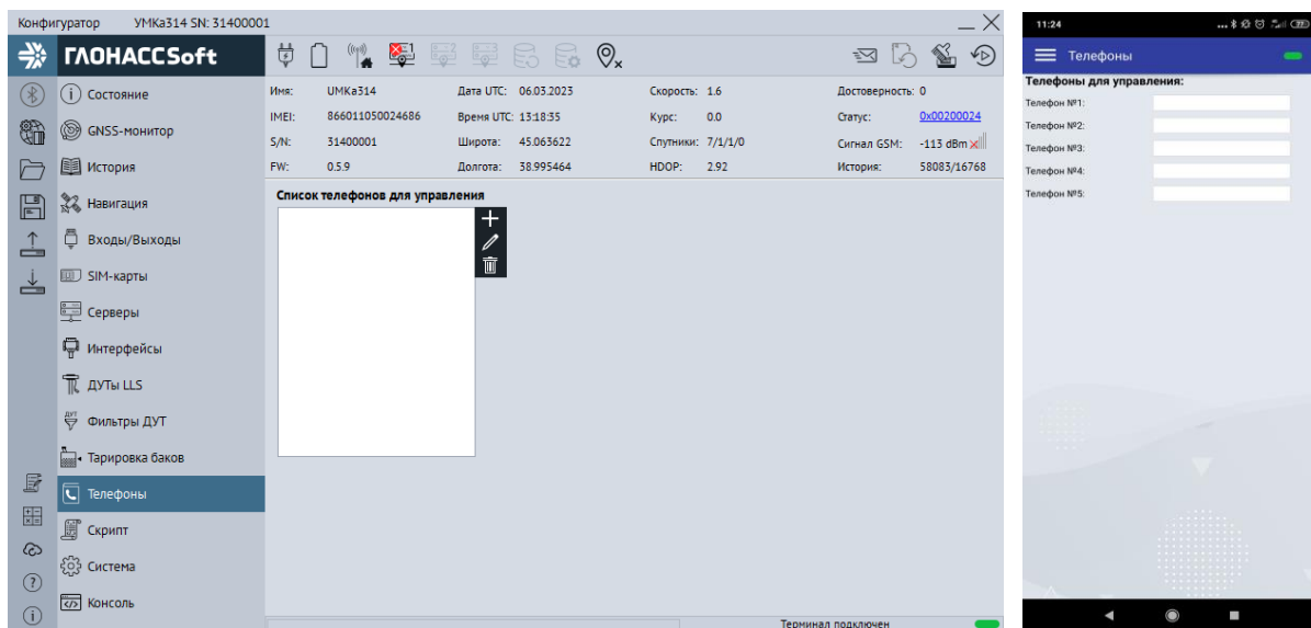
Рисунок 3.39 Вкладка «Телефоны»
