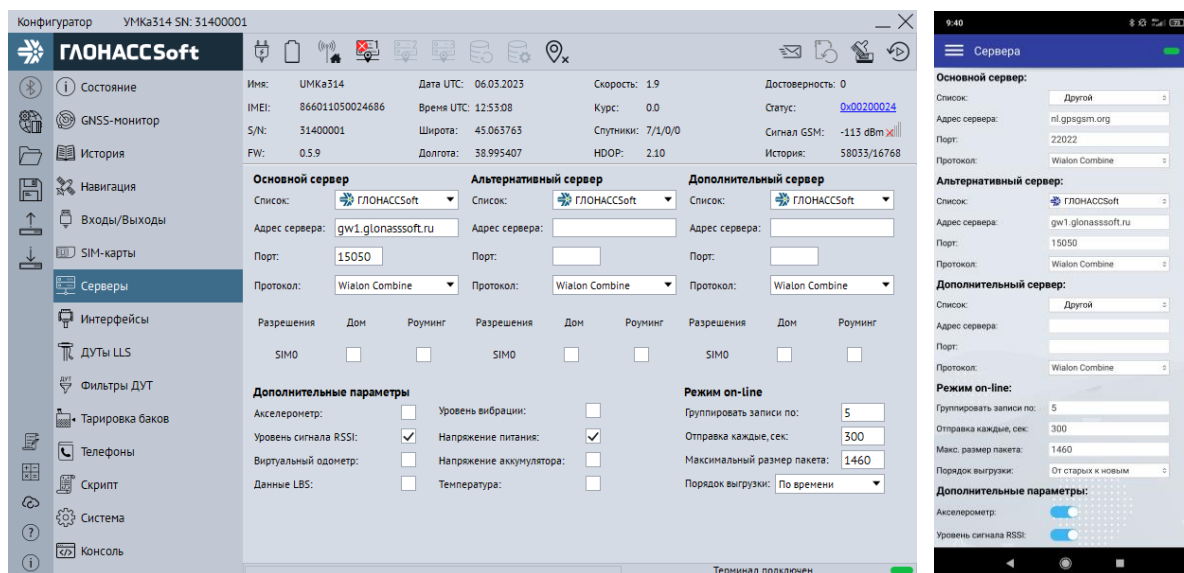
Рисунок 3.35 Вкладка «Серверы»
