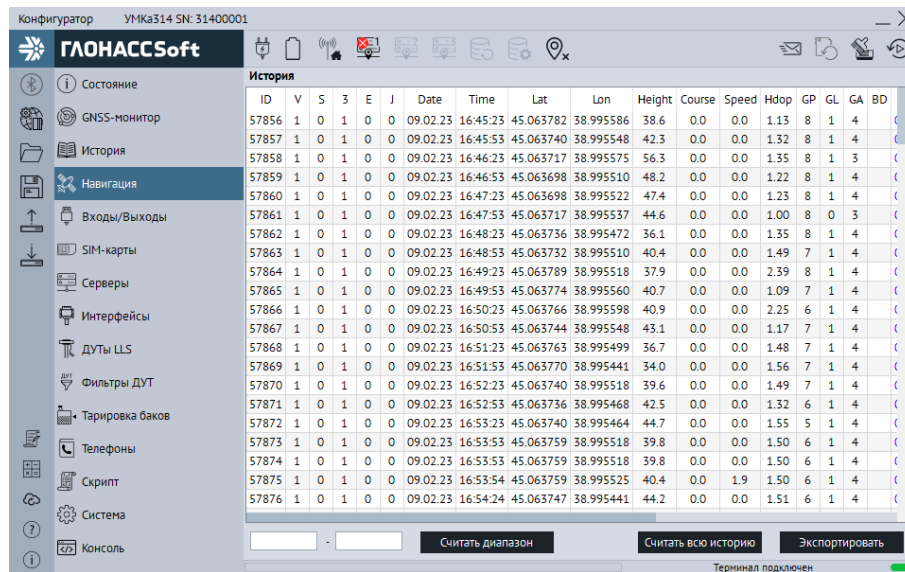
Рисунок 3.30 Вкладка «История»
