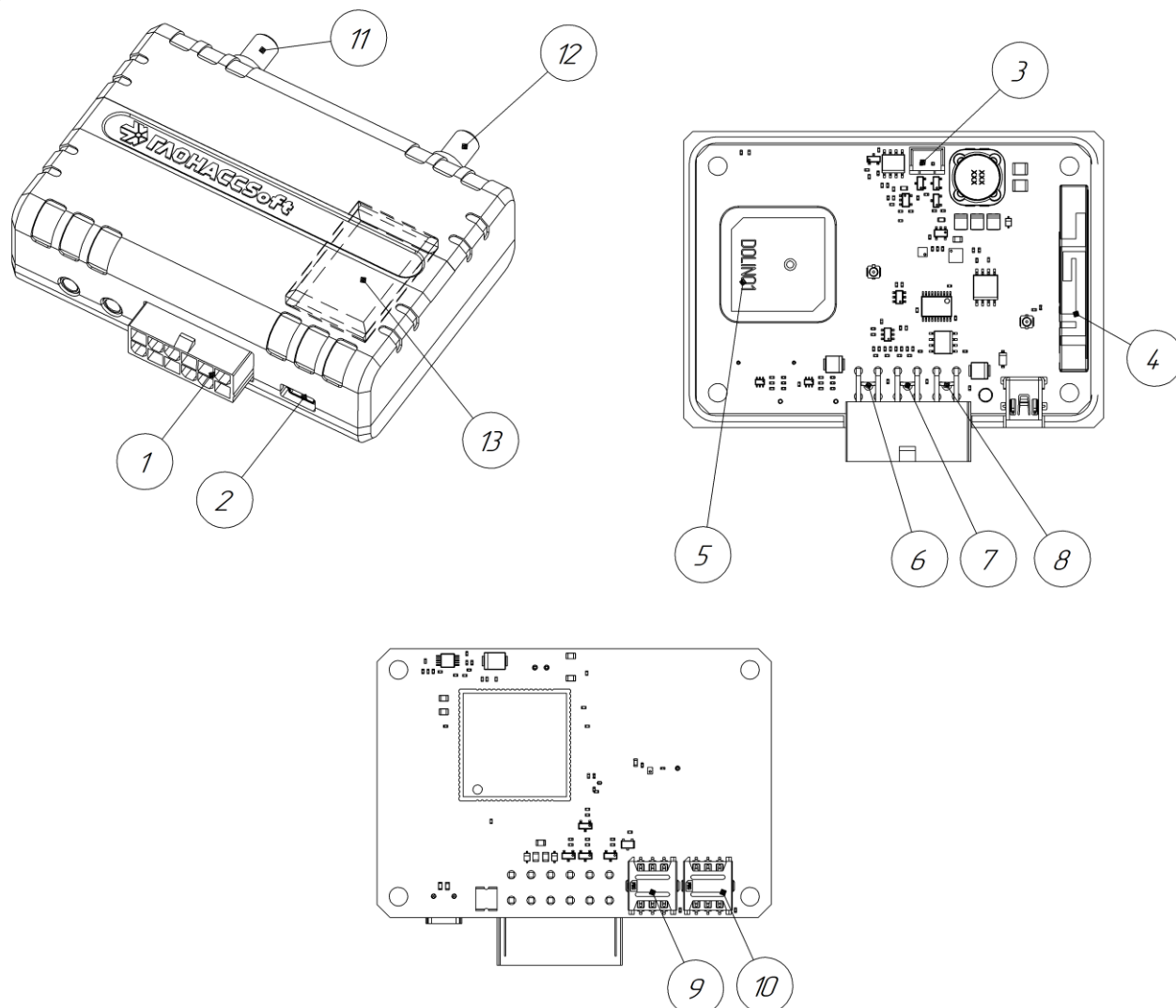
Рисунок 2.1 Основные элементы терминала УМКа314
