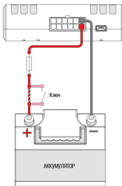
Рисунок 2.6 Подключение питания
