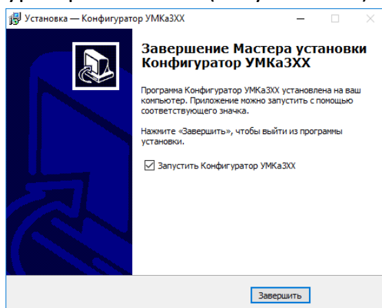
Рисунок 3.21 Запуск приложения
