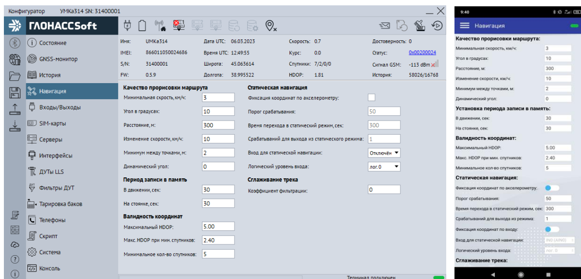
Рисунок 3.31 Вкладка «Навигация»
