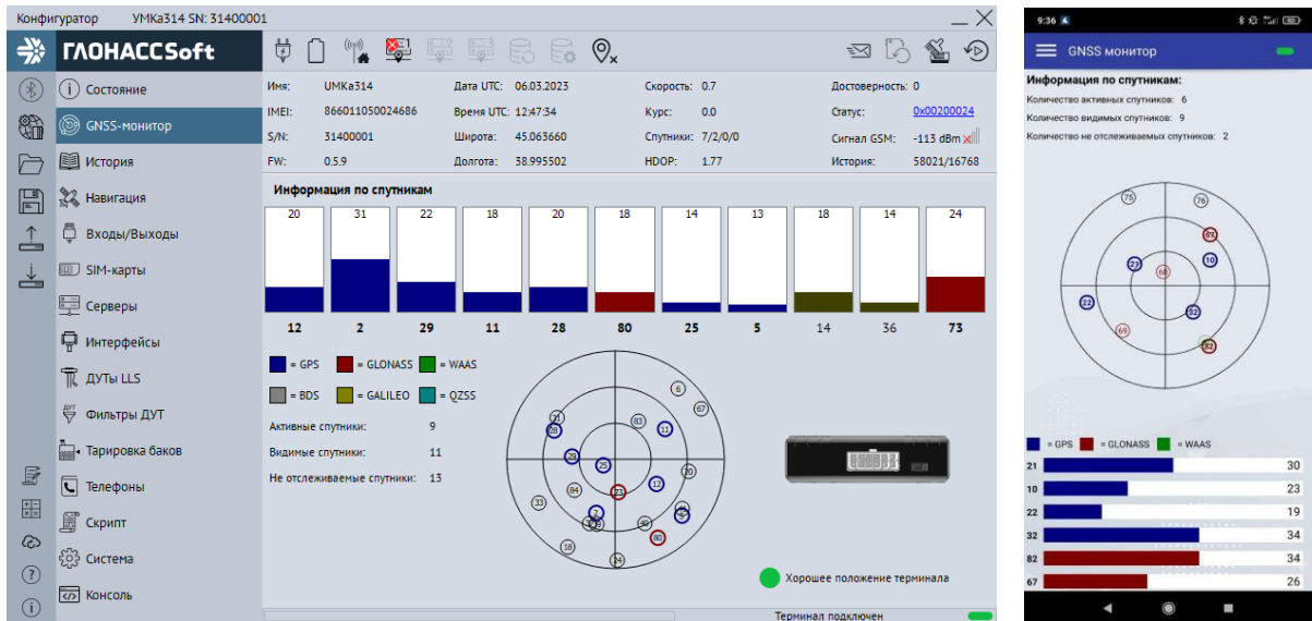
Рисунок 3.29 Вкладка «GNSS-монитор»
