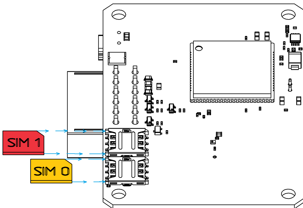
Рисунок 2.4 Установка SIM-карт
