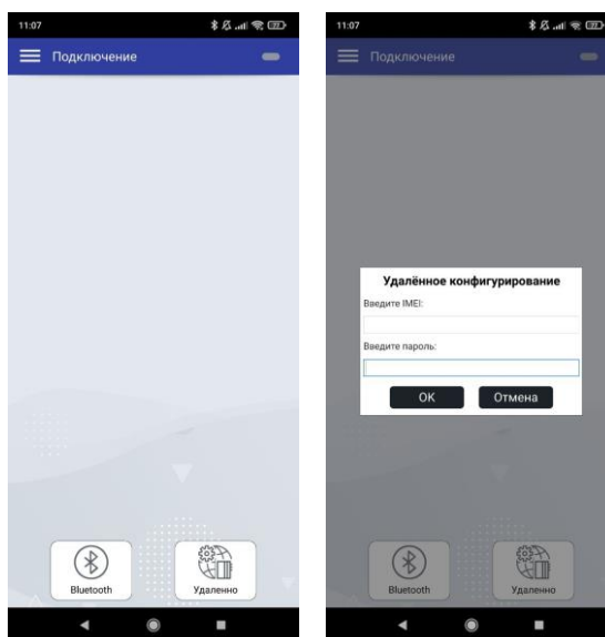
Рисунок 3.24 Список доступных терминалов
